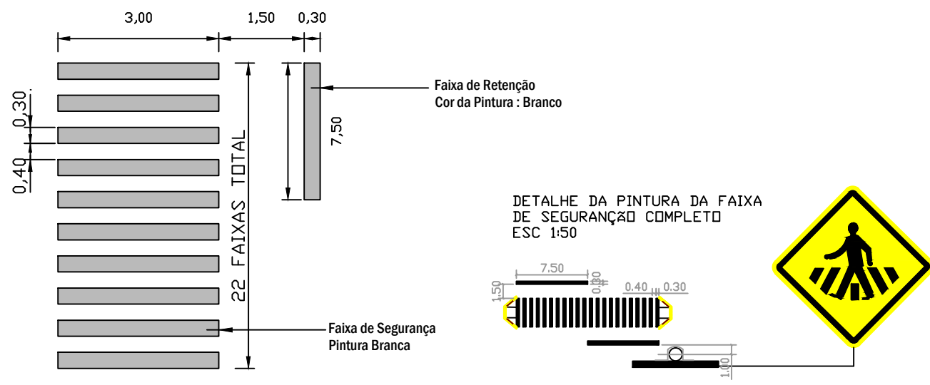
DETALHE DA FAIXA DE SEGURANÇA SEM ESCALA
